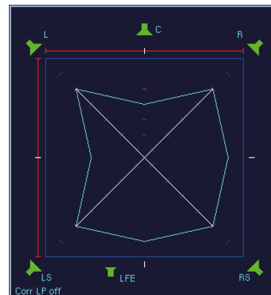
3 | Wie links, jedoch ist die Phase des linken Kanals um 180^\circ gedreht. Die Korrelation ist in den Kanalpaaren L - R und L - LS jeweils r = -1 , dort sind keine Phantomschallquellen ortbar.
