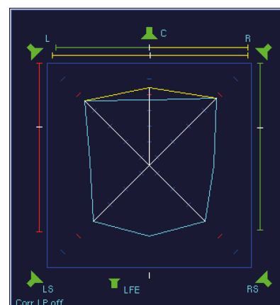
6 | Die ausgeknickte TVI-Linie zwischen LS und RS, keine Ausdehnung der PSI-Linie und Korrelation r = +1 in der unteren Korrelationsgradanzeige deuten auf ein identisches Mono-Signal in beiden Surroundkanälen hin.
