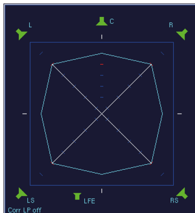
2 | Identisches Sinus-Signal mit gleichen Pegeln in den Kanälen L, R, LS, RS. Die Korrelation ist jeweils r = +1 (ausgeknickte TVI-Linien), Phantomschallquellen (PSI) genau mittig, ähnlich einem Mono-Signal.
