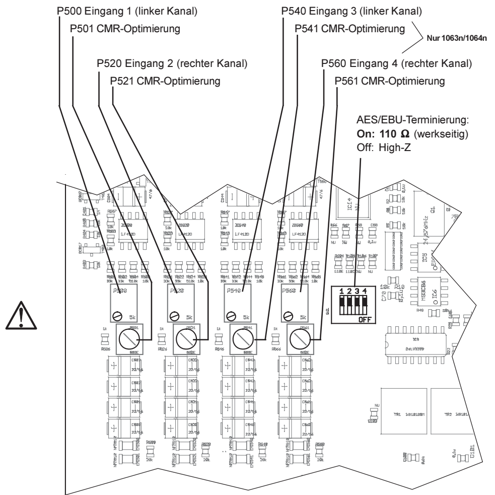
Bild 4-1 Teilansicht der Eingangsplatine
